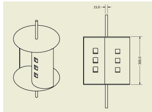
Gambar 2. Model Turbin Angin yang diteliti
